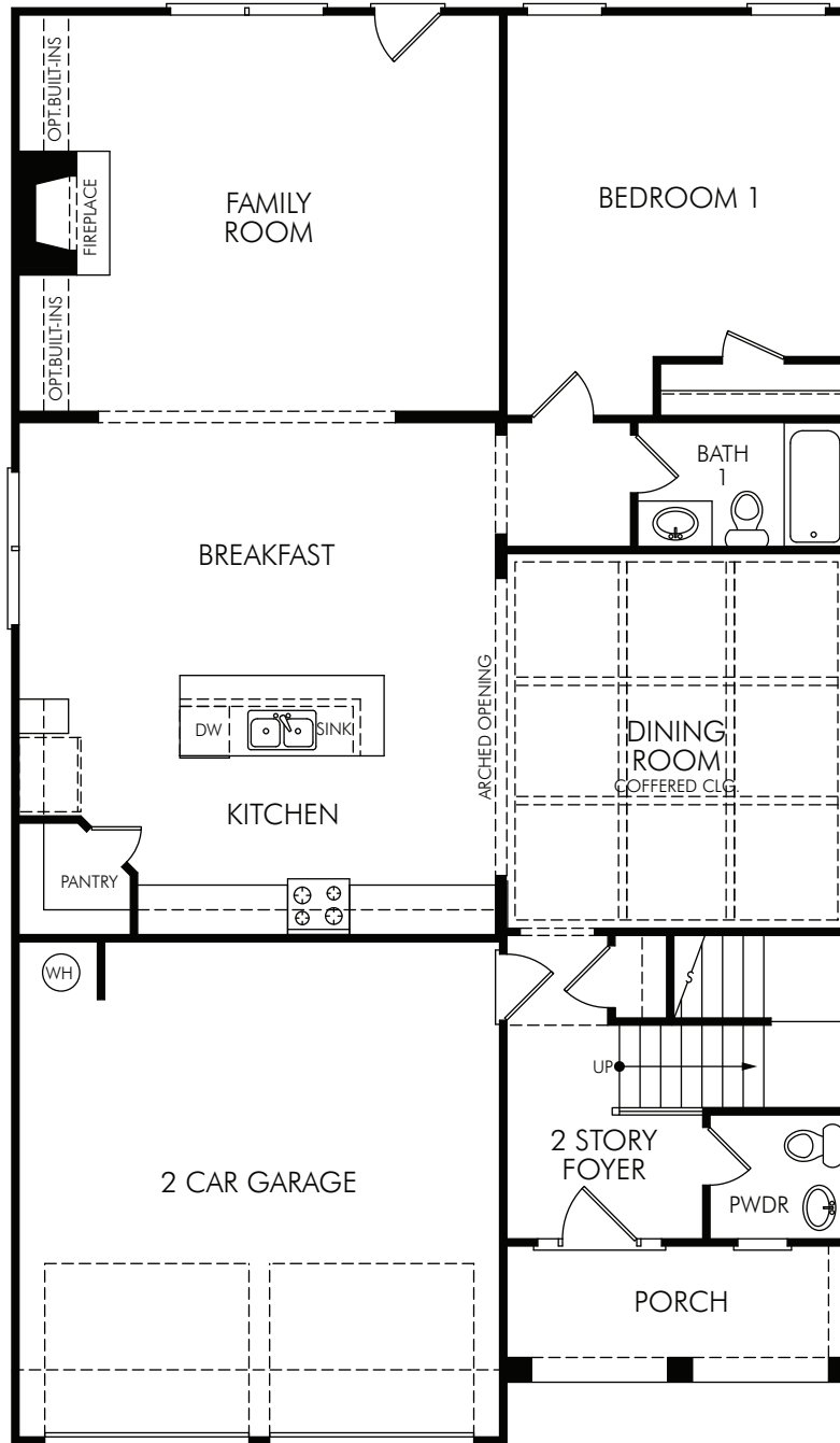
FIRST FLOOR OPTION 1-A
